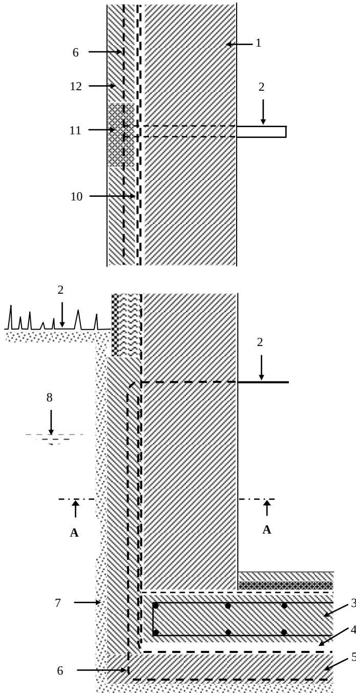
Şekil-L.7 Bina temeli yalıtım malzemesi içinde kalan temel topraklayıcının yerleştirilmesine örnek
