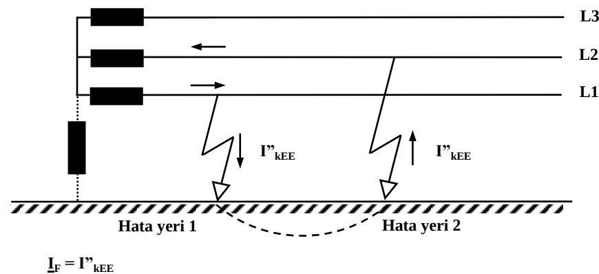
Şekil-4e Yıldız noktası yalıtılmış veya toprak teması kompanze edilmiş bir şebekede çift toprak temas akımı
