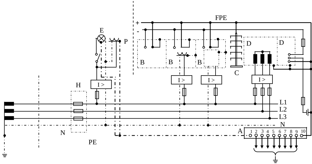
Şekil-19 Madde 21-c1'de belirtilen bir iletişim tesisinin fonksiyon ve koruma topraklamasına örnek (Not: Bu şekil mecburi olmayıp, yalnızca bir fikir vermek amacıyla taşımaktadır.)
