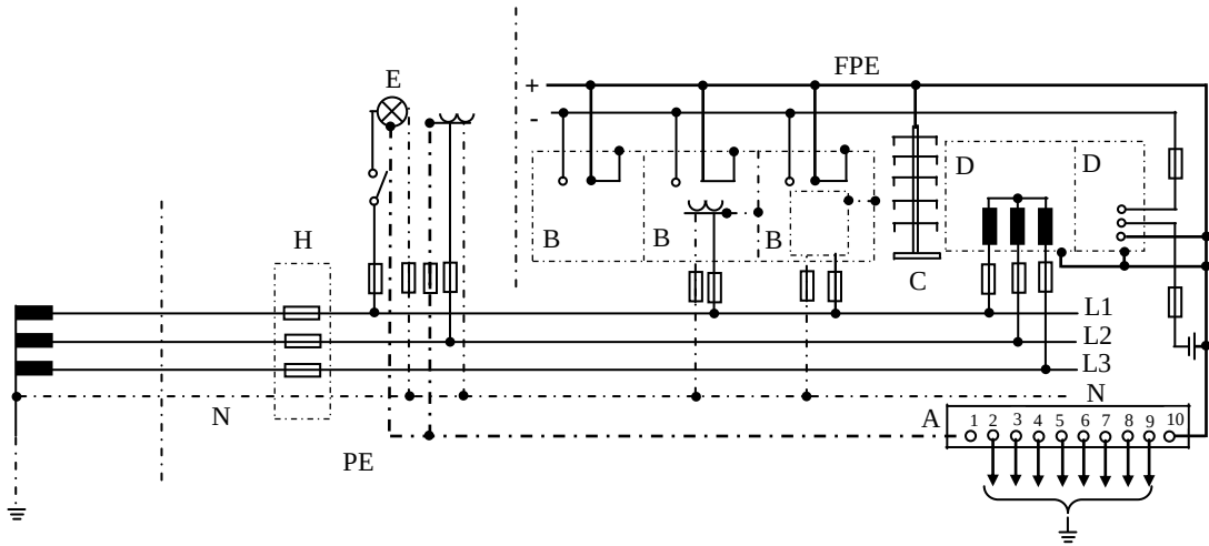
Şekil-20 Madde 21-c2'de belirtilen bir iletişim tesisinin fonksiyon ve koruma topraklamasına örnek (Not: Bu şekil mecburi olmayıp, yalnızca bir fikir vermek amacıyla taşımaktadır.)
